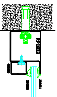
隔声墙体与其他结构墙体连接
